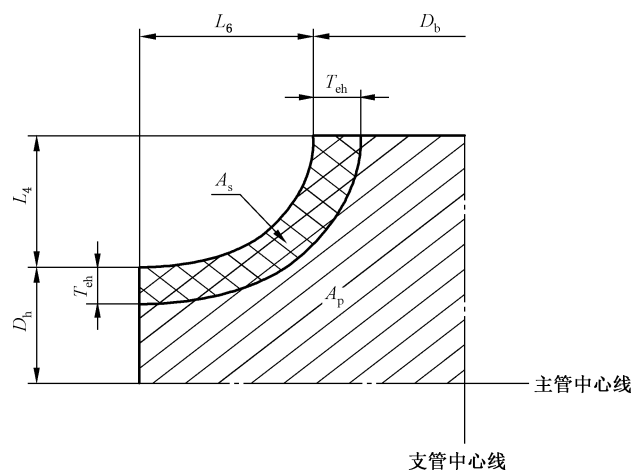
图 L.1 三通补强计算示意图
