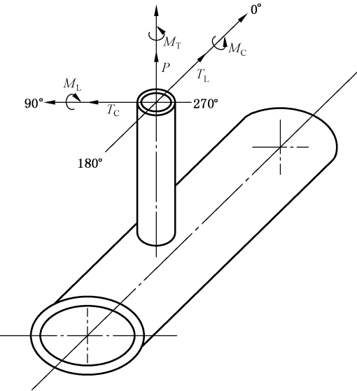
图 O.1 设备管口承受的力和力矩方向
