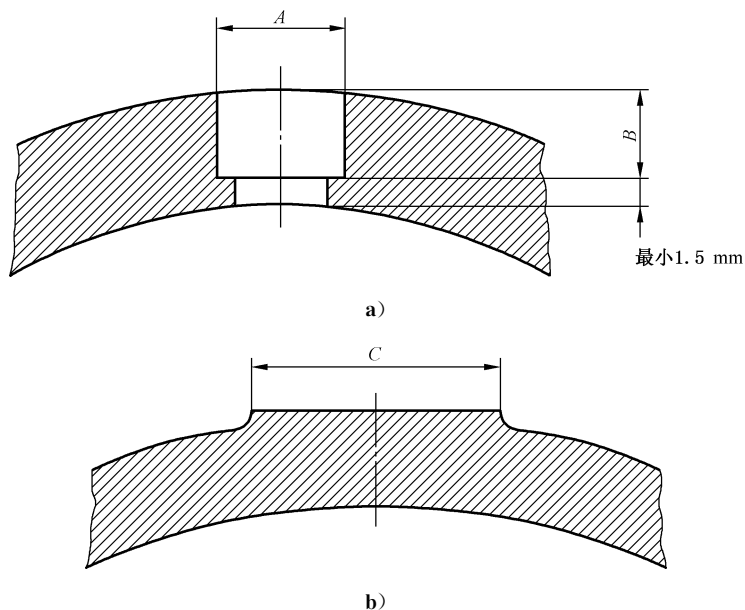
图 4 承口和凸缘示意图
