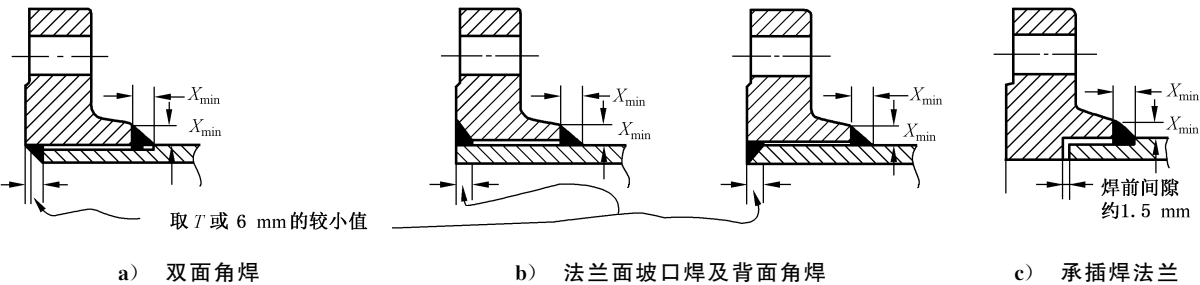
标引符号说明： T ——直管名义厚度； X_{min} ——角焊缝最小焊脚尺寸。
